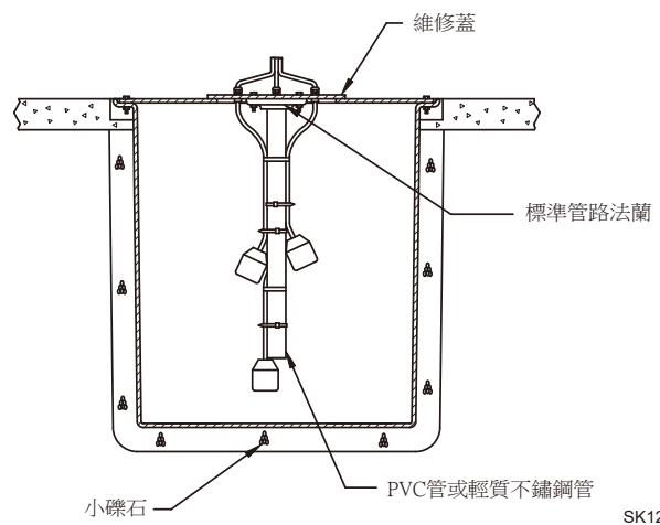
鋼蓋板水池上標準浮子安裝桿
